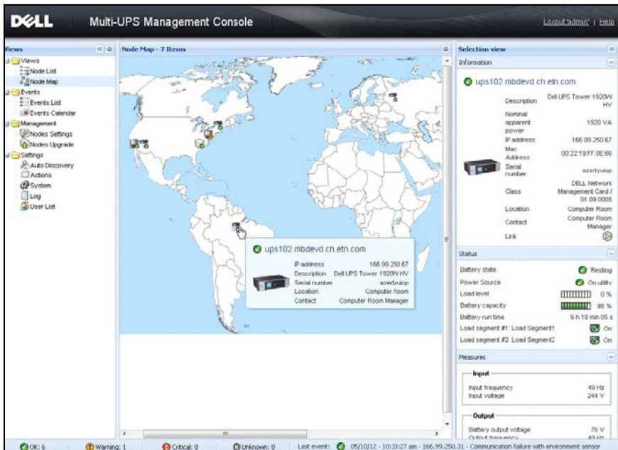
Schéma 1. MUMC DellPage principale
