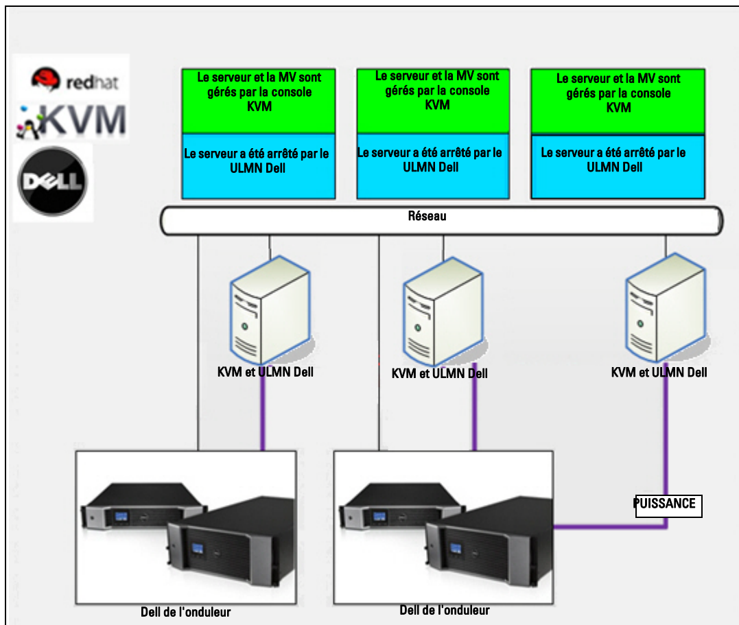
Schéma 60. ULMN Dell Configurations pour Red Hat KVM ou OpenSource KVM
