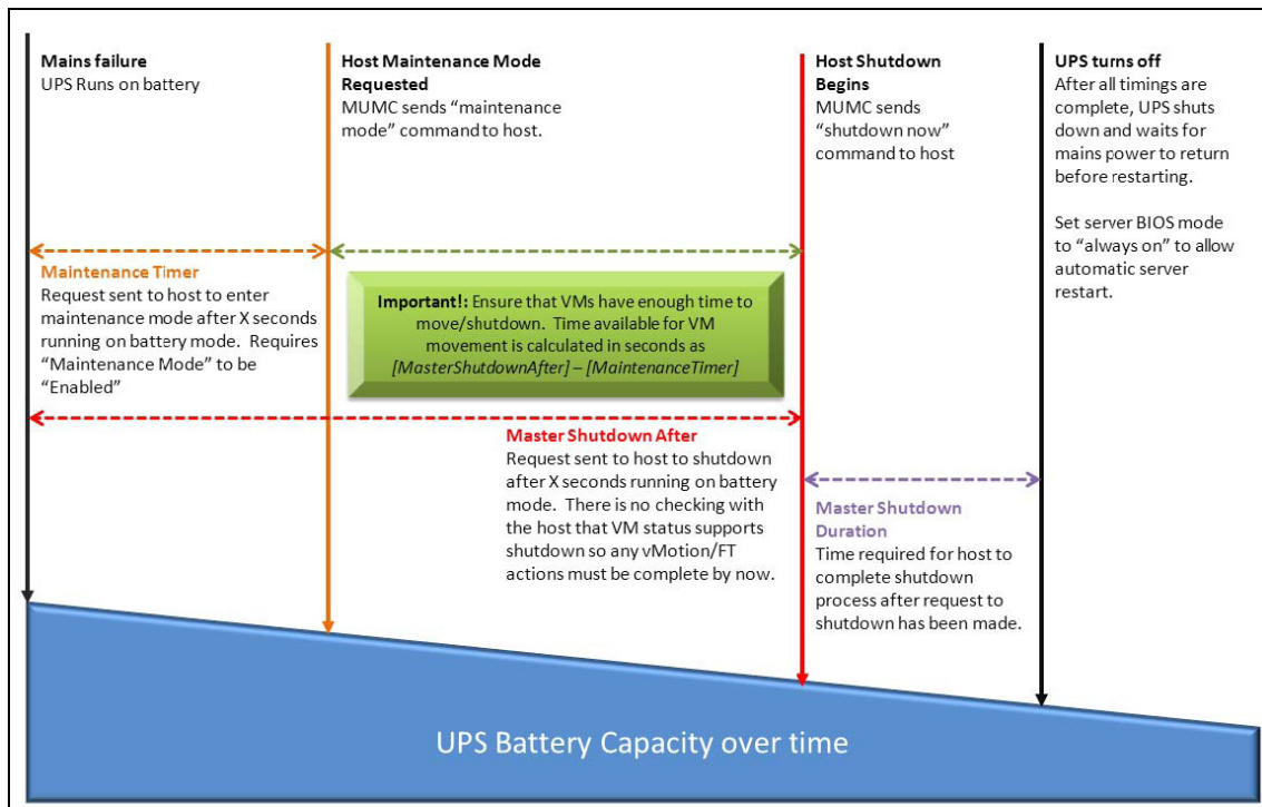
Schéma 73. Capacité de la batterie de l'onduleur à long terme
