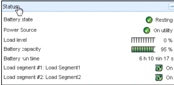
Schéma 20. Panneau relatif à l'état
