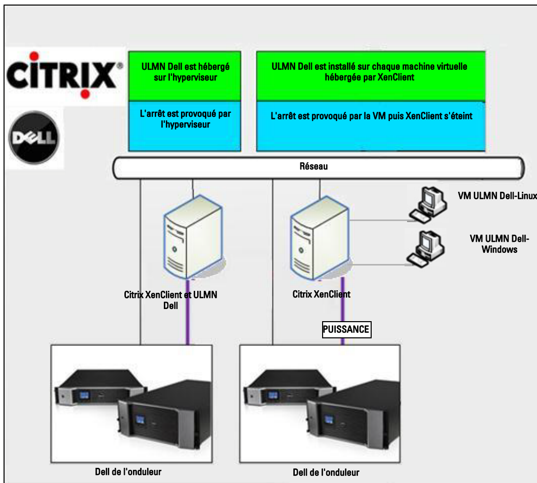
Schéma 61. ULMN Dell Configuration pour XenClient
