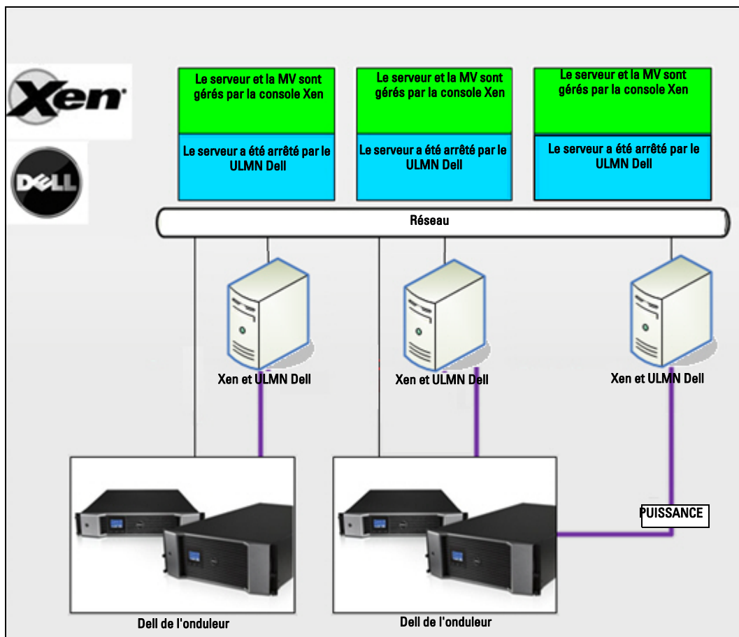
Schéma 59. ULMN Dell Configurations pour OpenSource Xen
