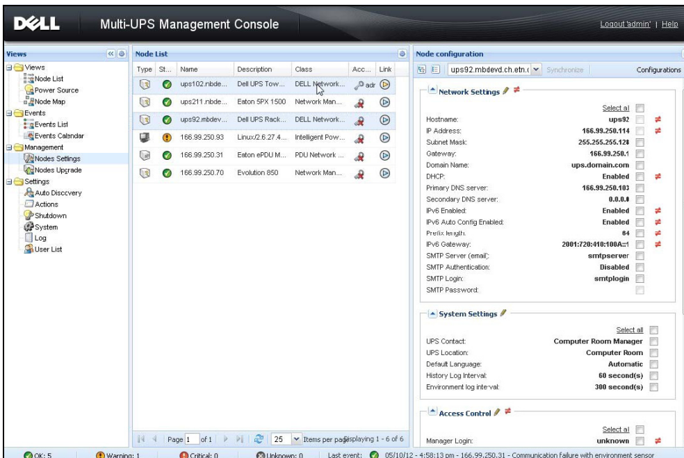
Schéma 52. Configuration de masse NMC
