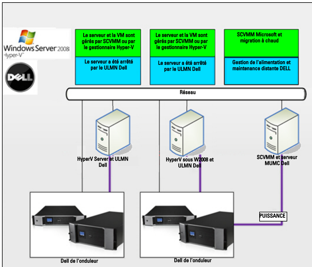
Schéma 57. ULMN Dell et configuration MUMC Dell pour HyperV
