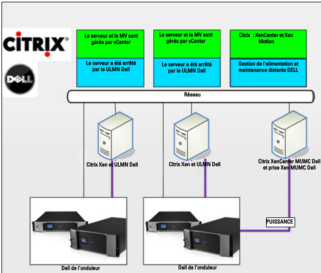
Schéma 58. ULMN Dell et configuration MUMC Dell pour XenServer
