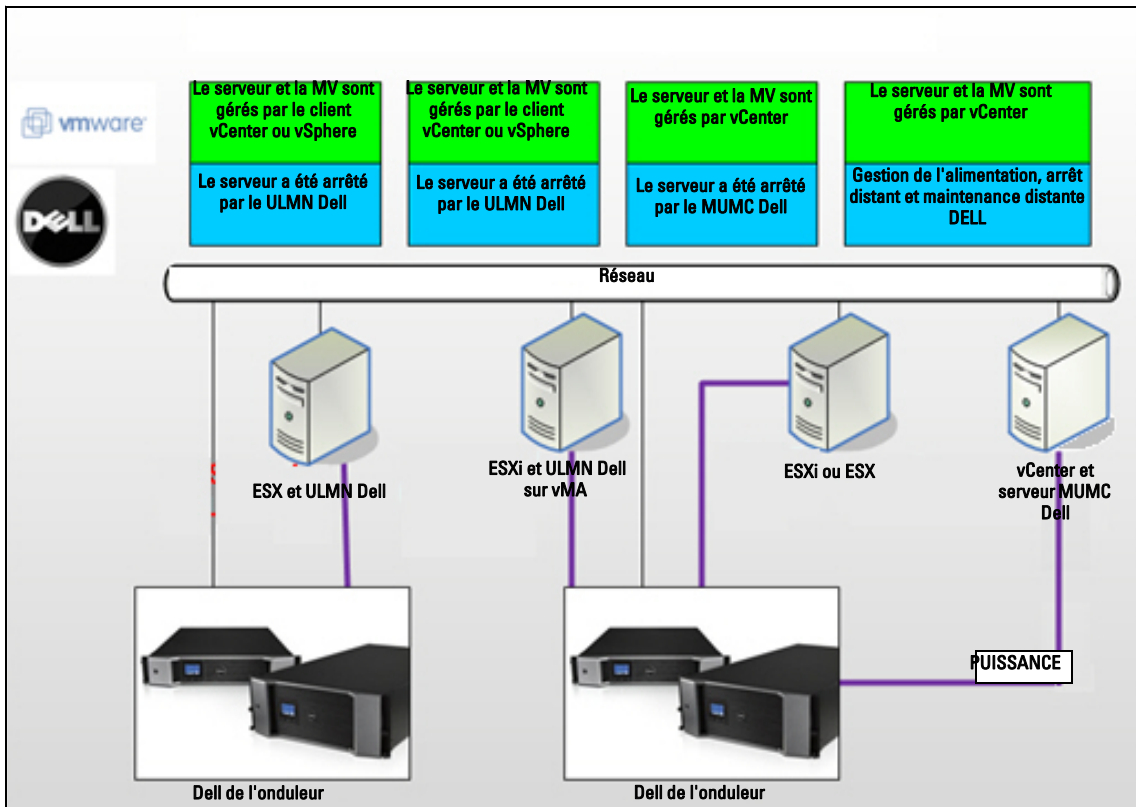
Schéma 56. ULMN Dell et configuration MUMC Dell pour VMware
