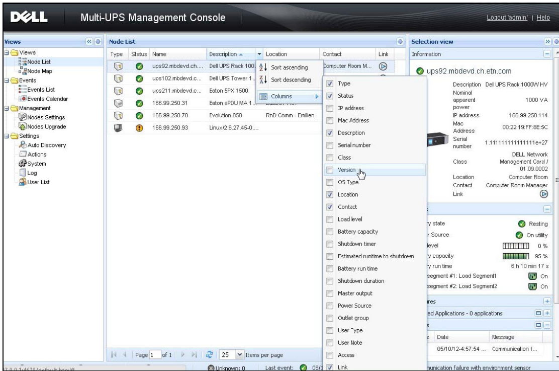
Schéma 17. Ajouter des colonnes dans l'aperçu de la liste de nœuds
