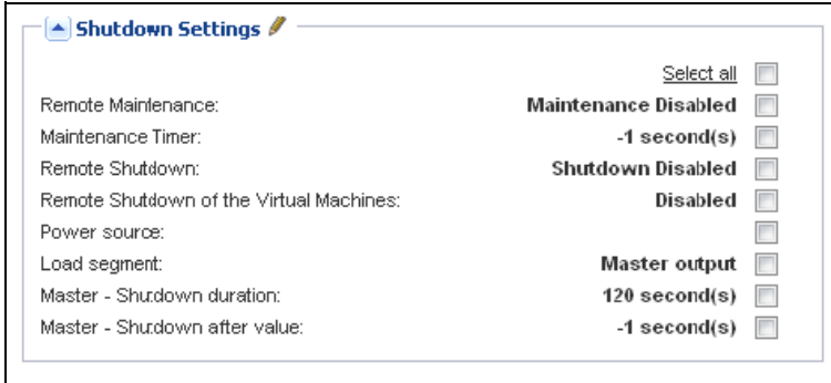
Schéma 71. Paramètres d'arrêt de vCenter et SCVMM - Avant la configuration
