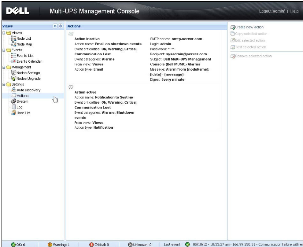
Schéma 7. Page relative aux actions
